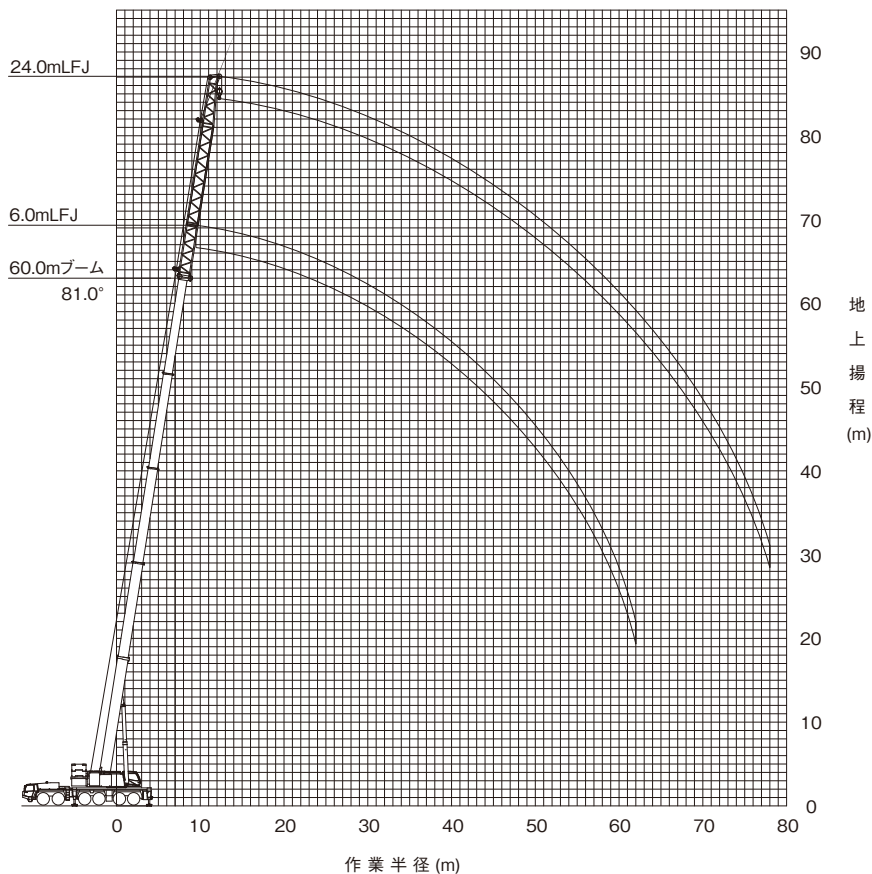
ブーム+フィックスジブ
