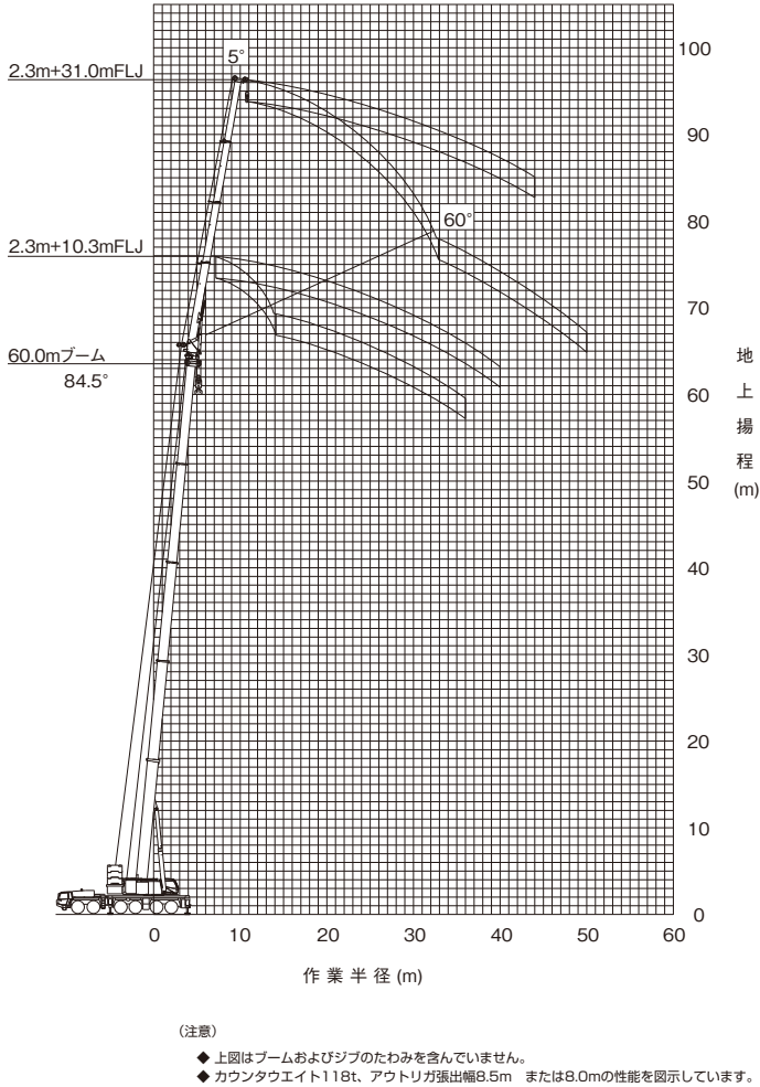
ブーム+フルオートラフingジブ
